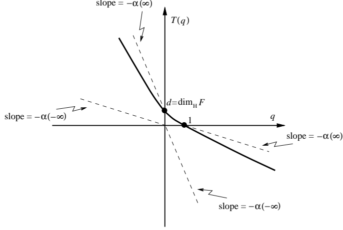
FIGURE 2A) T(q)
